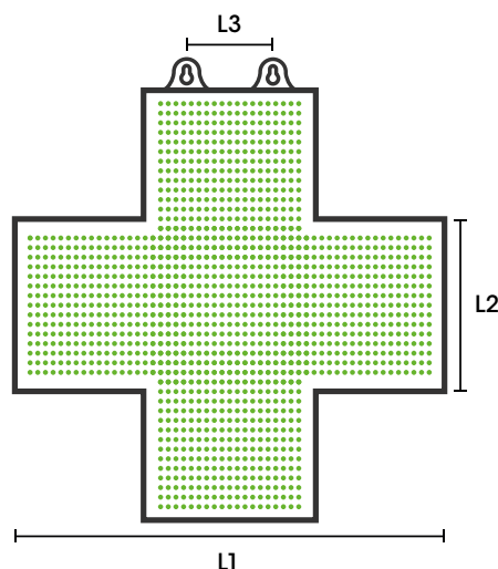
Face / Aanzicht (mm)
